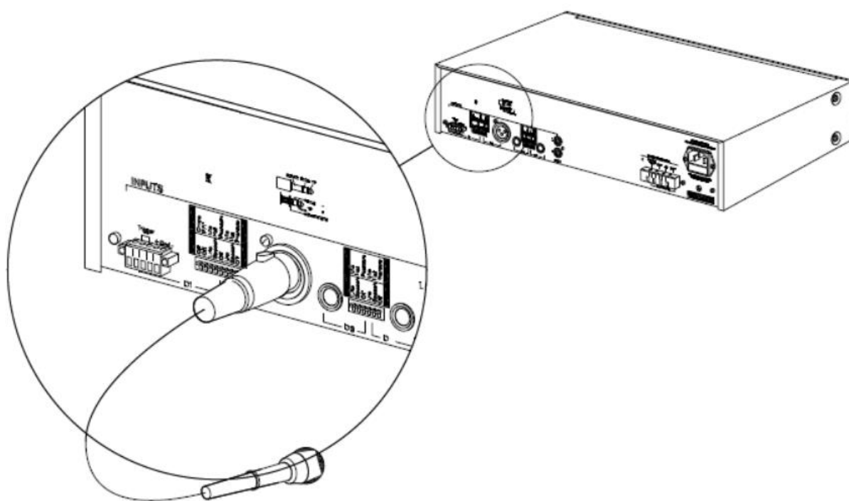
รูปที่ 4 การต่อใช้งานไมโครโฟนที่ input 2
